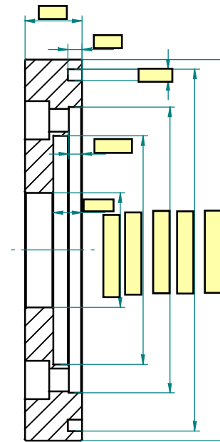
Schnitt A-A
