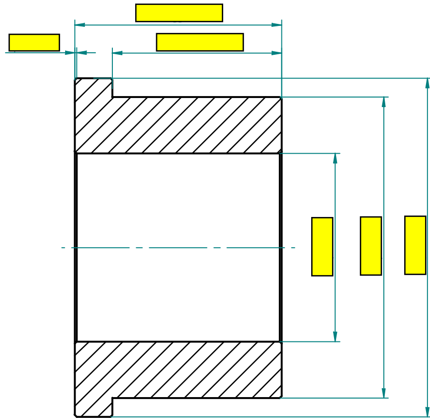
Schnitt A-A
